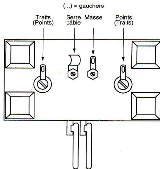
ETM-SQ vue de dessous et connexions.
